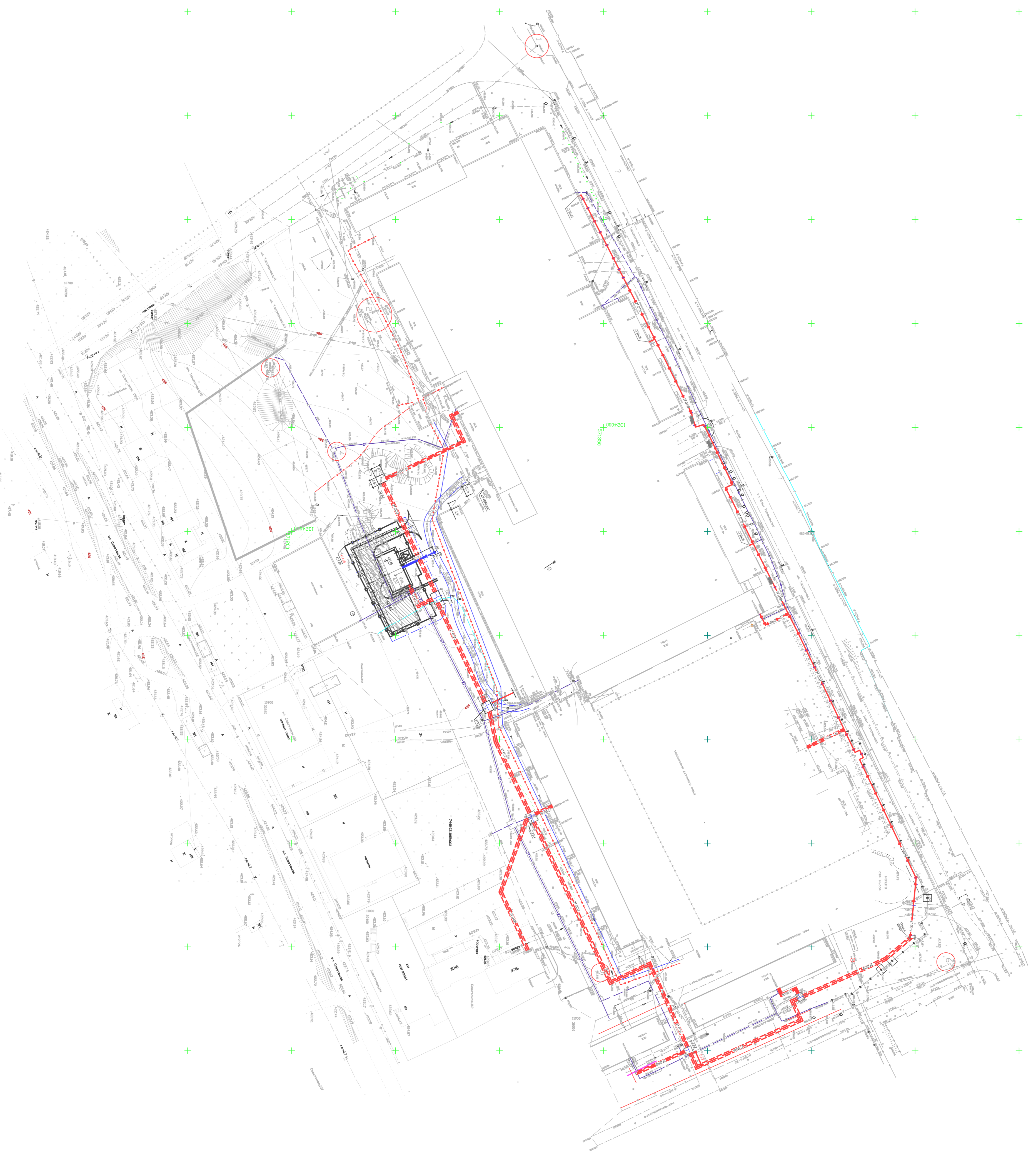
План сетей (1:1000)
